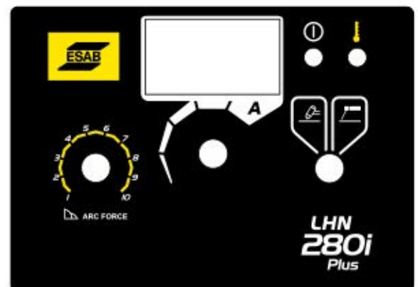
Panel LHN 280i Plus
